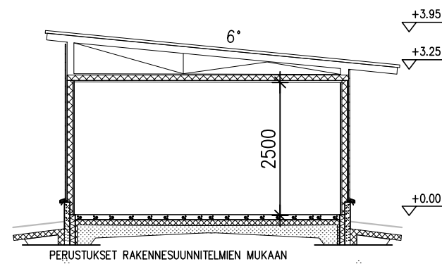
LEIKKAUS A-A
