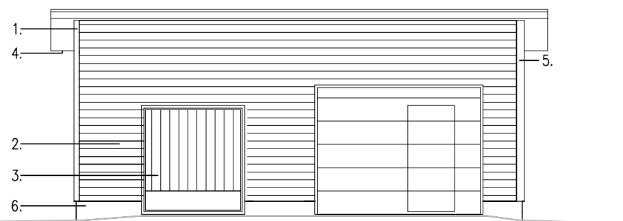
JULKISIVU LUOTEeseen
